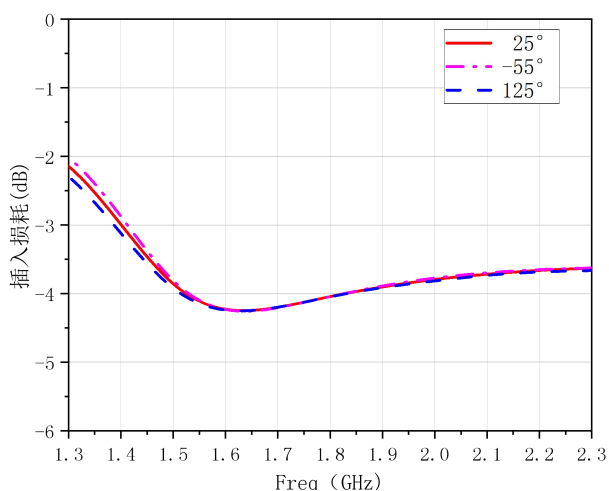
插入损耗 VS 温度
