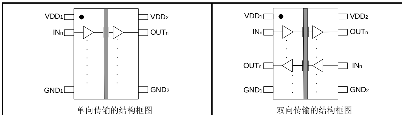
功能框图
