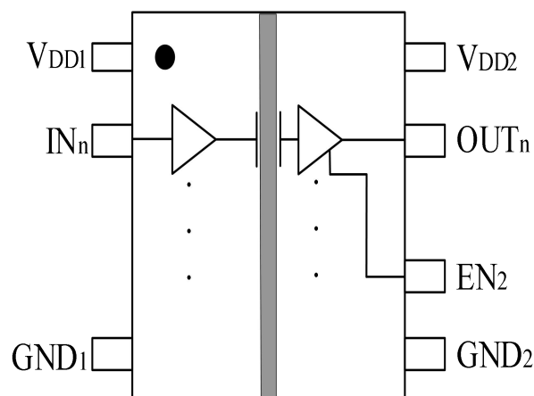
带单向使能端的单向传输的结构框图
