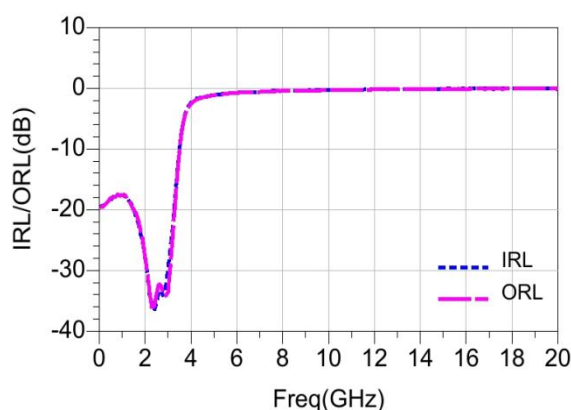
输入/输出回波损耗 VS 频率
