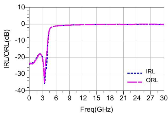
输入/输出回波损耗 VS 频率
