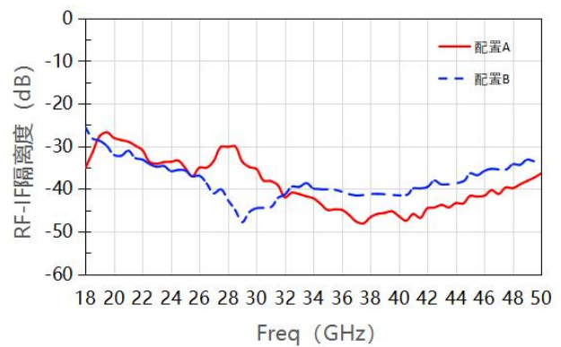
隔离度 RF-IF VS 频率
